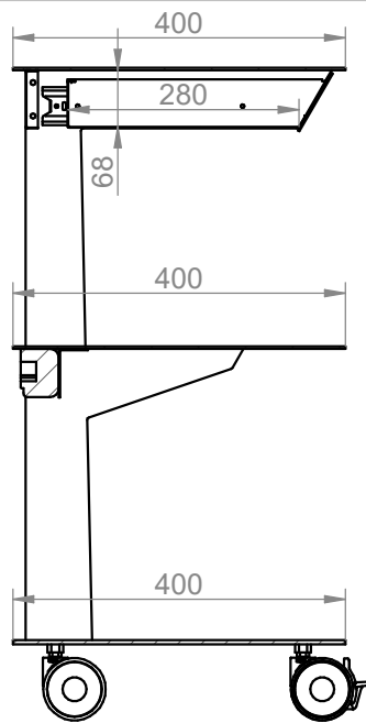
SEZ A-A
